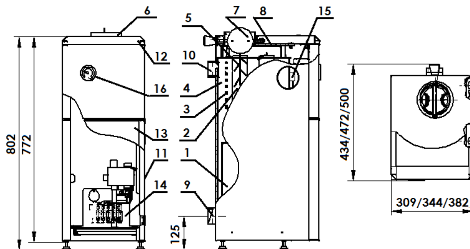
Рис.1. Котлы КСЦ-Г/ГВ-10/12/16...
